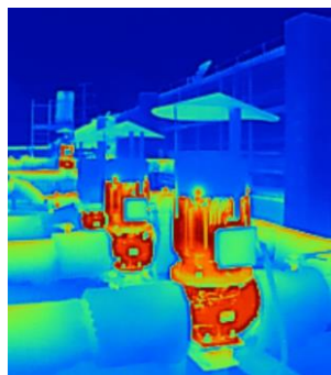
Motor
